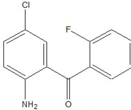
2-Amino-5-chloro-2'-flurobenzophenone
